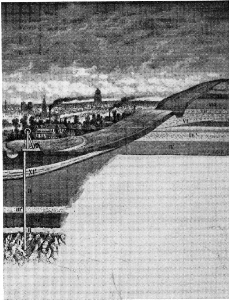
Schema van de HUIDIGE Brusselse ondergrond tot op 100 m. diepte (tot op de rotsen)
