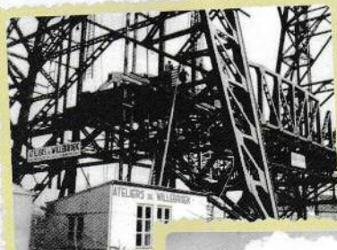
De brug tijdens de constructie in 1951-52.
